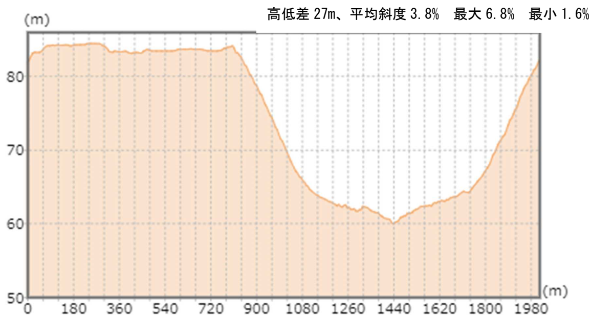
高低図
