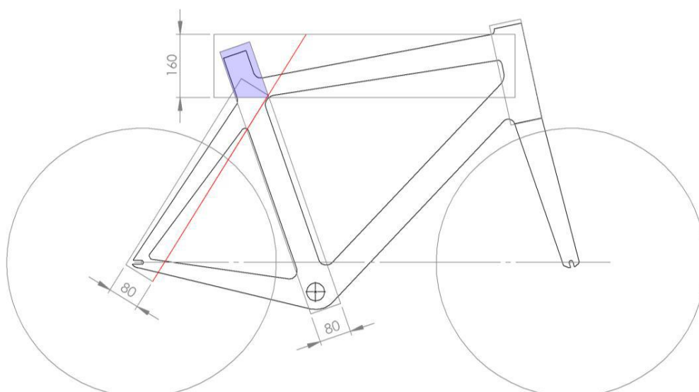
Figure 27: Illustration of the rule on the inclination of seat stays 図 27: シート・ステイの傾斜の規則の説明
