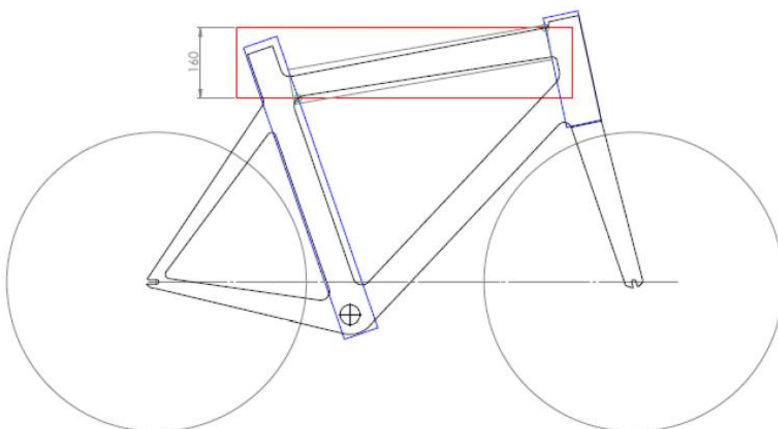
Figure 17: Illustration of maximum allowed sloping top tube 図 17: トップ・チューブの許容最大傾斜の説明
