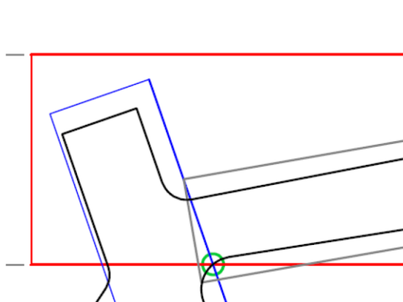
Figure 18: Lowest point (circled in green) that must be contained within the 16 cm high horizontal box 図 18: 最下点(緑の丸印)は 16cm 高の水平なボックスに含まなければならない
