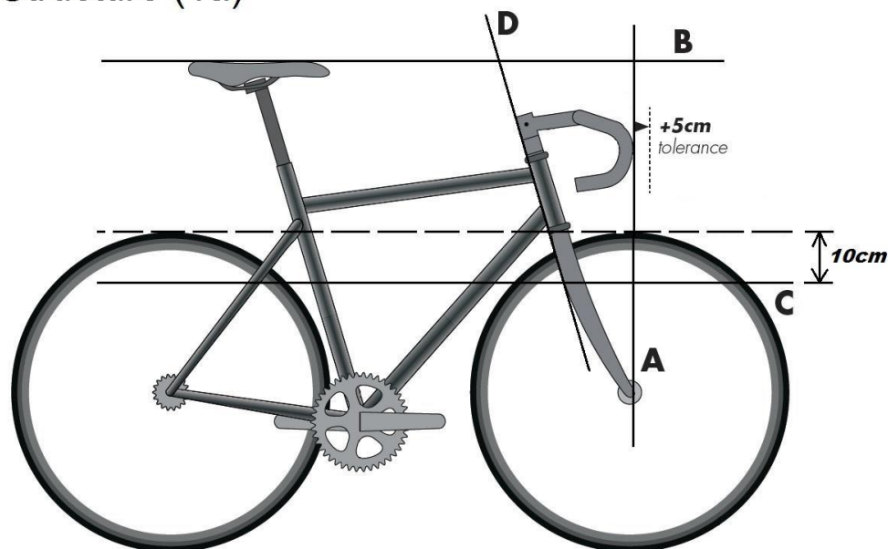
Structure (1a)
