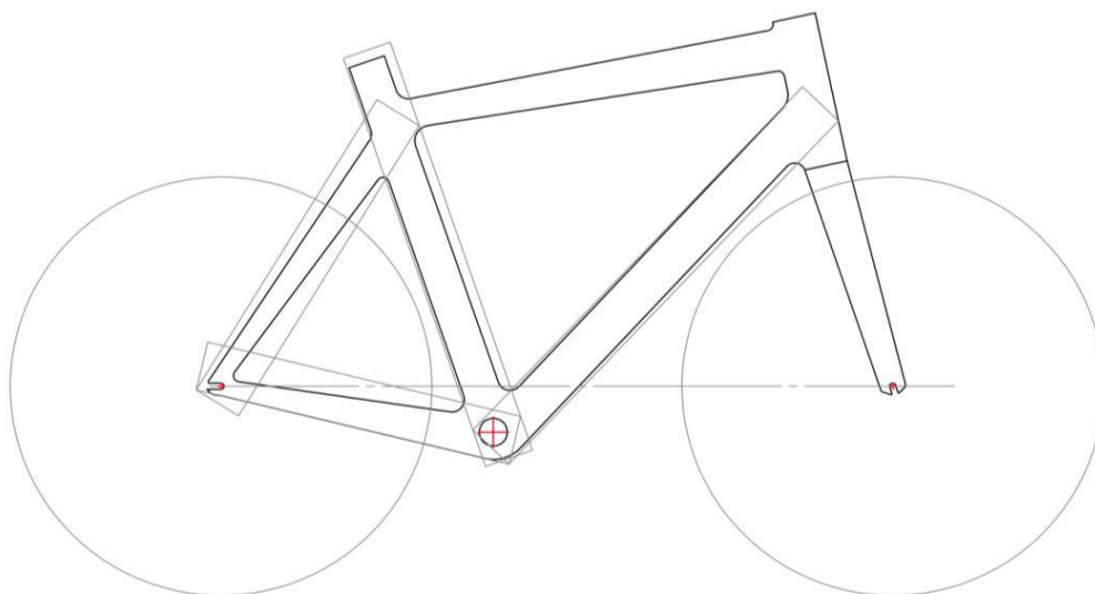
Figure 10: Illustration of the bottom bracket and rear wheel axles inside the corresponding boxes. 図 10: 対応するボックスの中のボトム・ブラケット軸と後車軸の説明。
